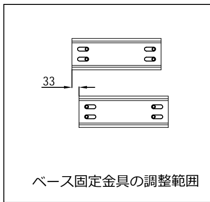
ベース固定金具
