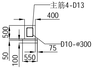
基礎詳細図
