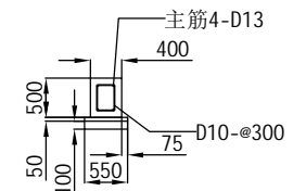
基礎詳細図
